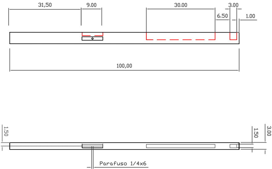
Espelho pé DIREITA (1x)
