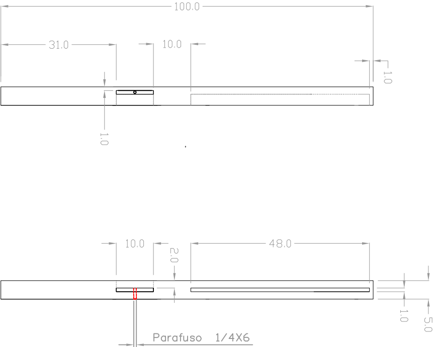
Espelho: pé (2x)
