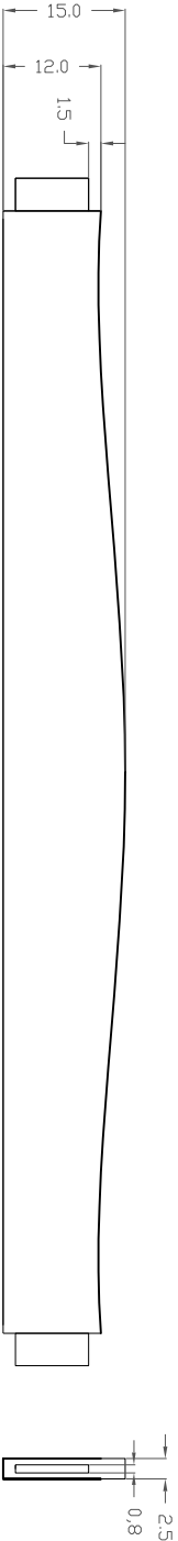
Peseira: peça longitudinal (1x)
