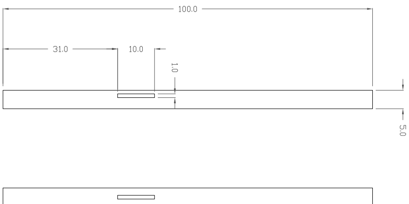
Espeelho: pé (2x)
