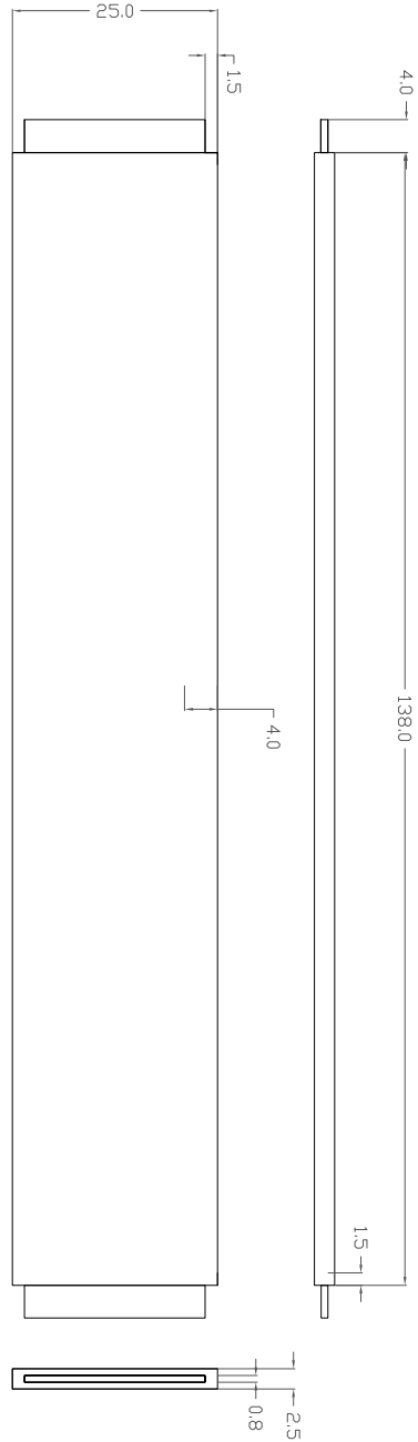
Espelho : peça longitudinal 4 (1x)
