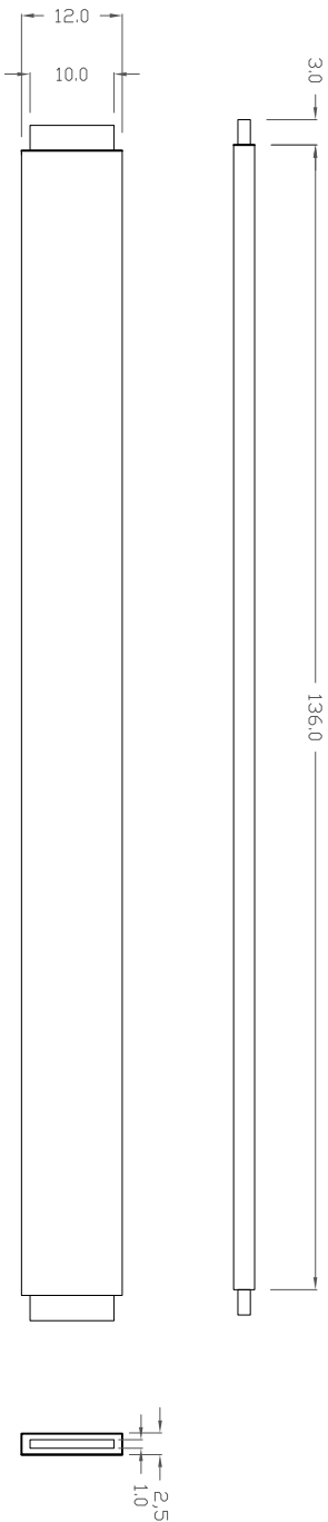
Espelho e peseira: peça longitudinal (2x)
