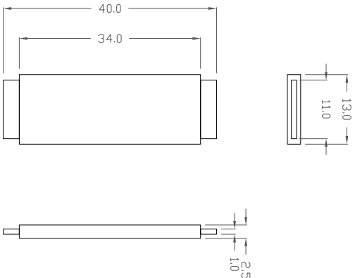
Espelho: peça transversal 6 (1x)
