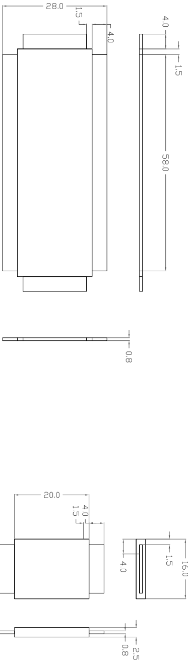
Espelho : peça longitudinal 2 (2x) (base arumã)
