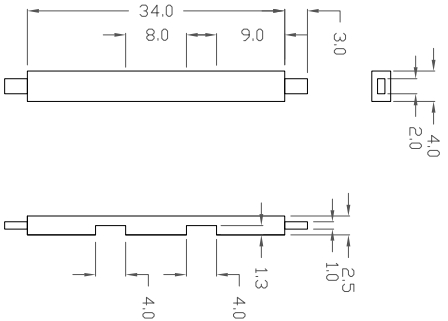
Espelho: peça transversal 5 (4x)
