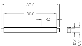
Espelho: peça transversal 4 (4x)
