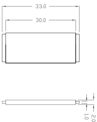
Espelho: peça transversal 2 (1x)
