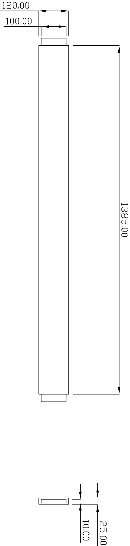
TRAVESSA ESPELHO
