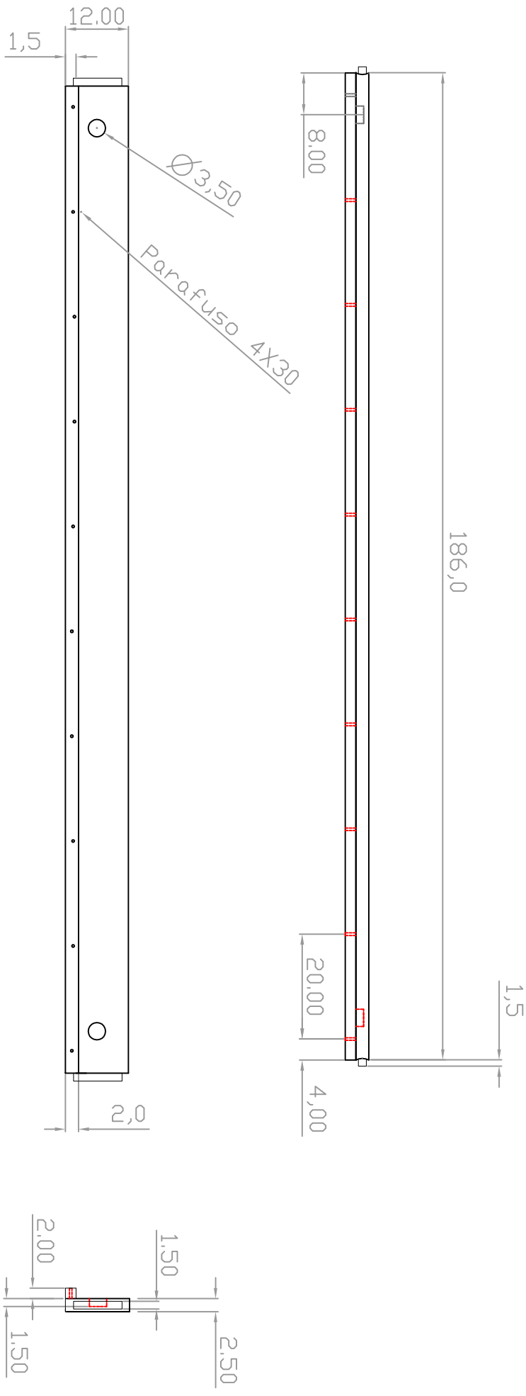
Lateral e apoio do estrado (2x)
