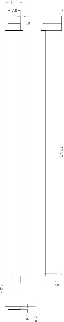
Espelho : peça longitudinal 1 (1x)
