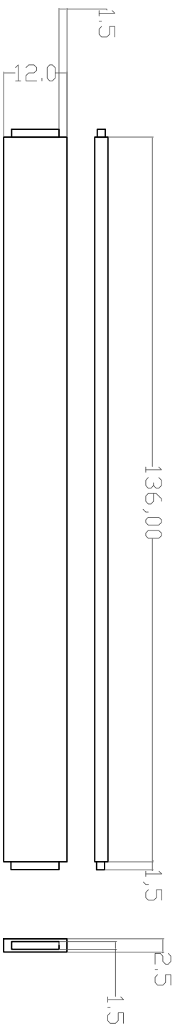
Espelho peça longitudinal 2 (1x)
