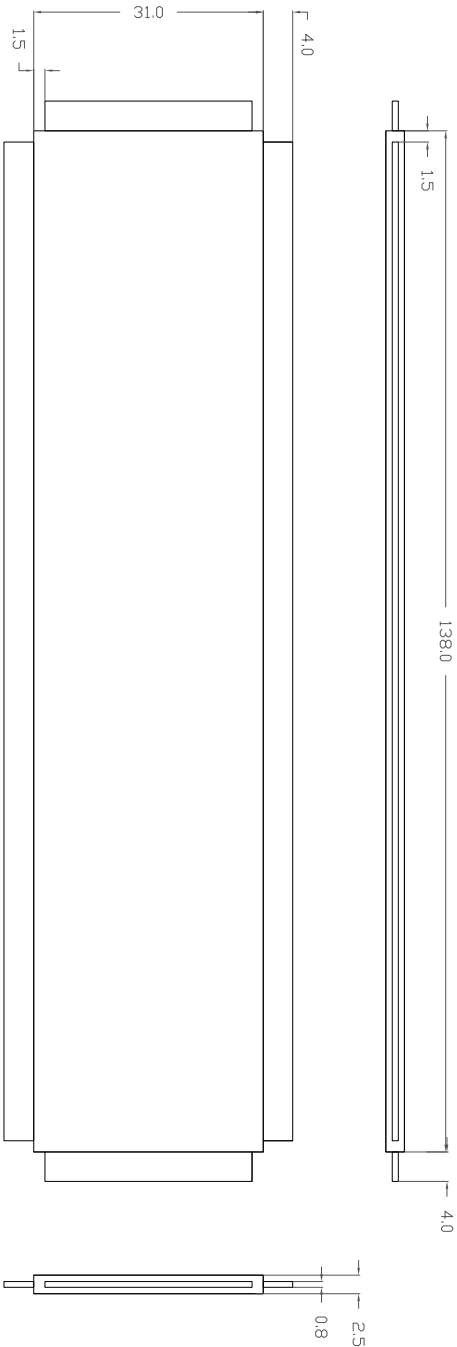
Peseira: peça longitudinal 2 (1x)
