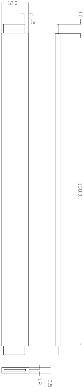
Espelho: peça longitudinal 5 (1x)
