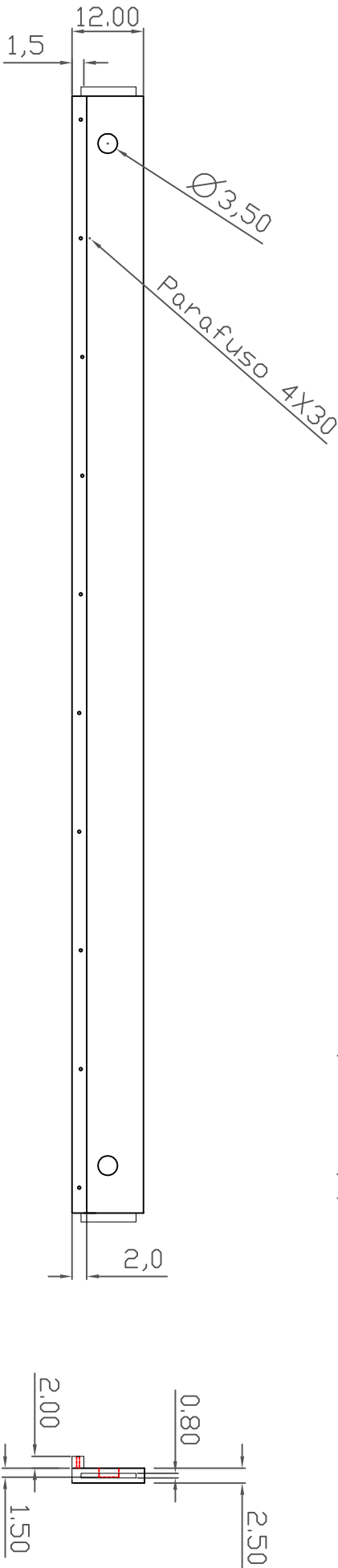
Lateral e apoio do estrado (2x)
