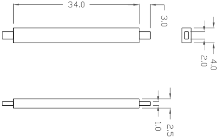
Espelho: peça transversal 4 (4x)
