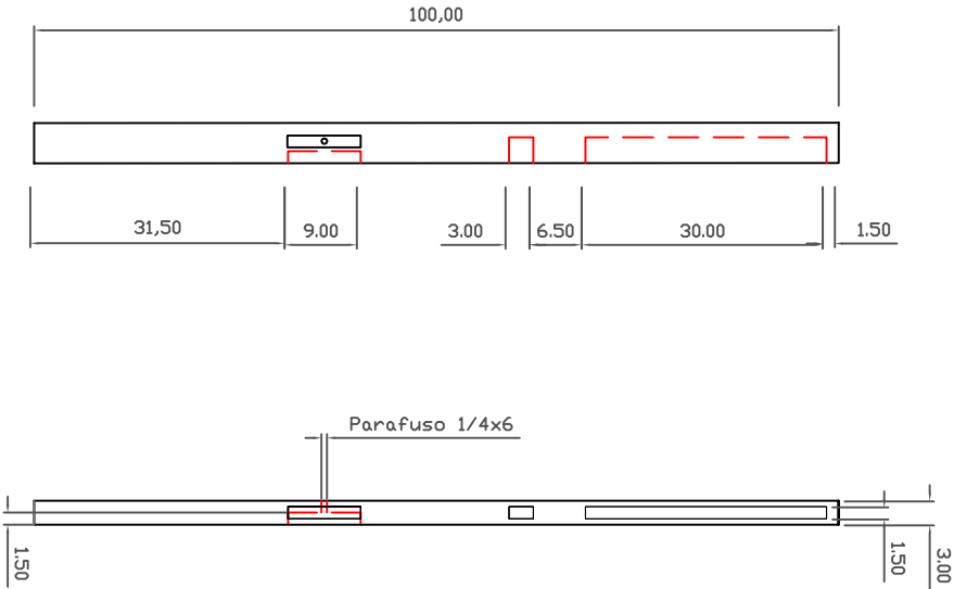
Espelho pé ESQUERDA (1x)
