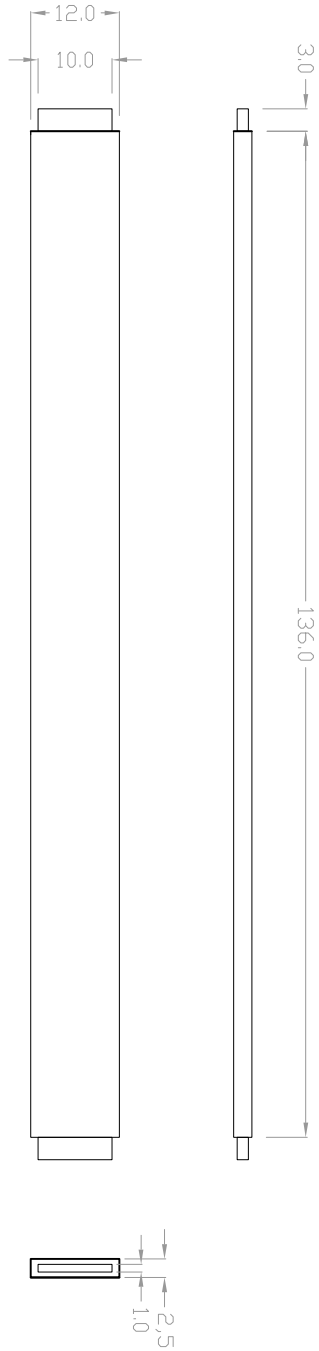
Espelho e peseira: peça longitudinal2 (2x)
